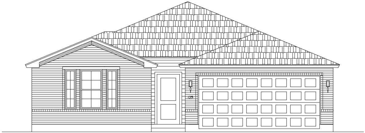
ELEVATION A
