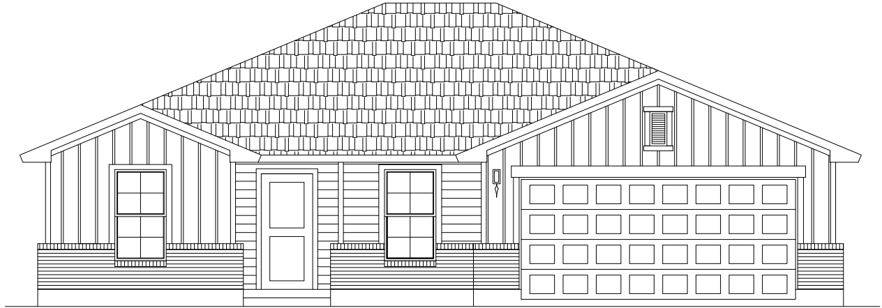
ELEVATION N
