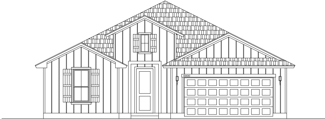
ELEVATION A
