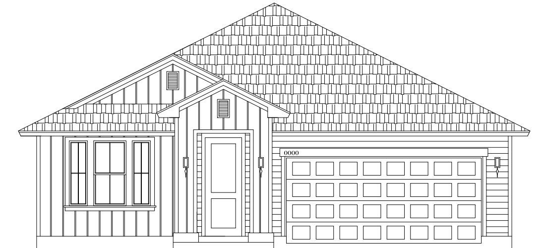
ELEVATION B
