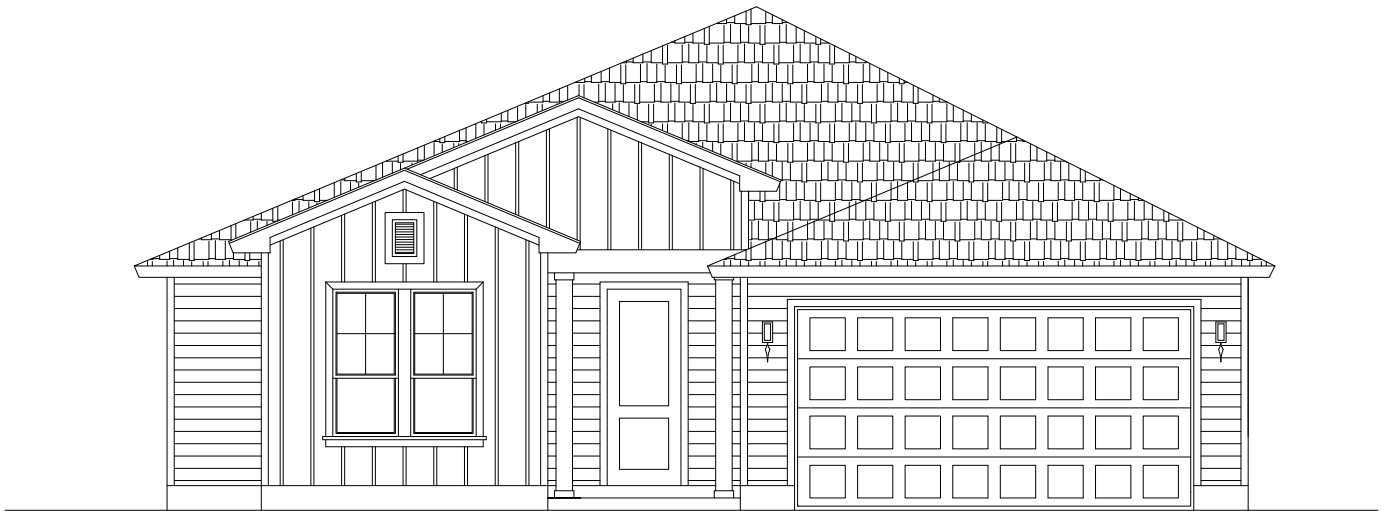
ELEVATION A
