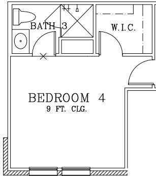
OPTIONAL BEDROOM 4
